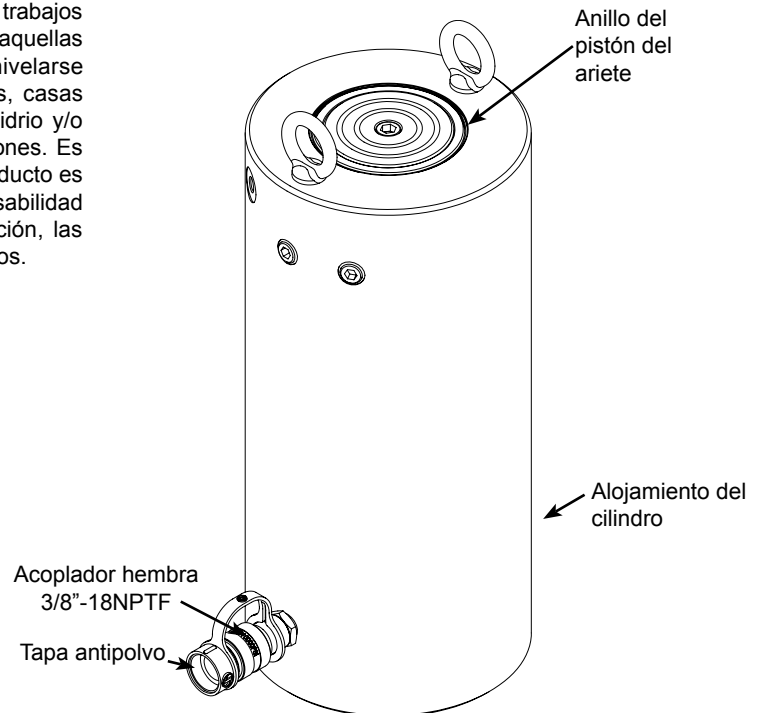
Figura 1: Componentes habituales del cilindro
